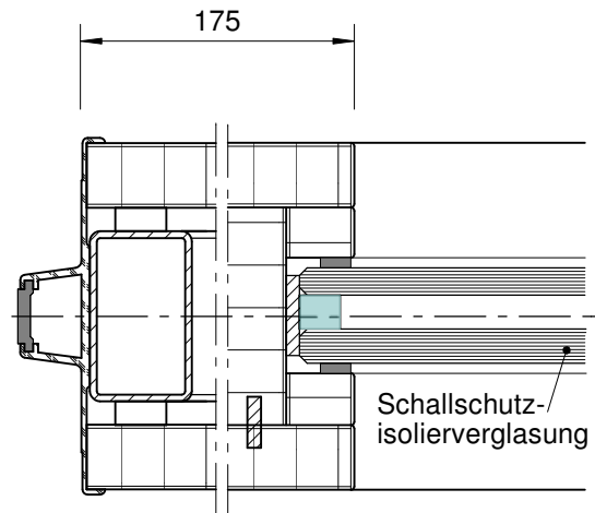
Element mit Schallschutzisolierverglasung Typ Topas
