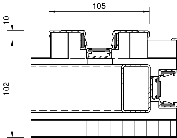
Element mit Seitenanschluss Typ Topas
