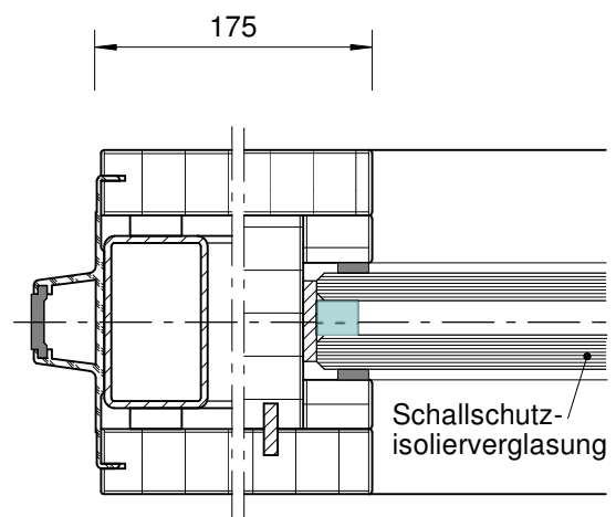
Element mit Schallschutzisolierverglasung Typ Karat
