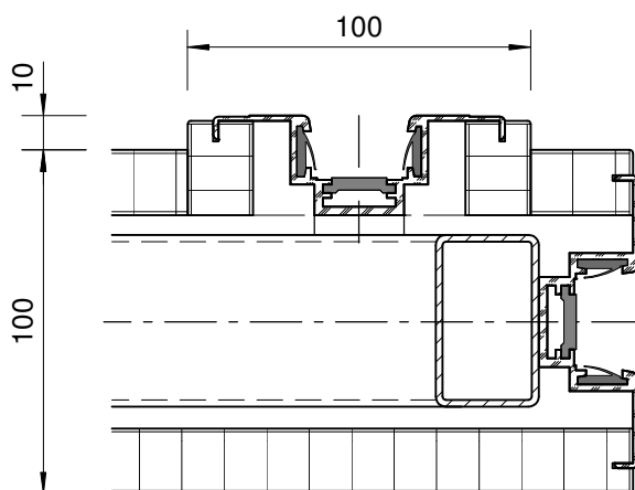
Element mit Seitenanschluss Typ Karat
