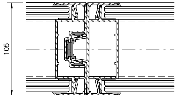
Elementverbindung Vollglaselemente
